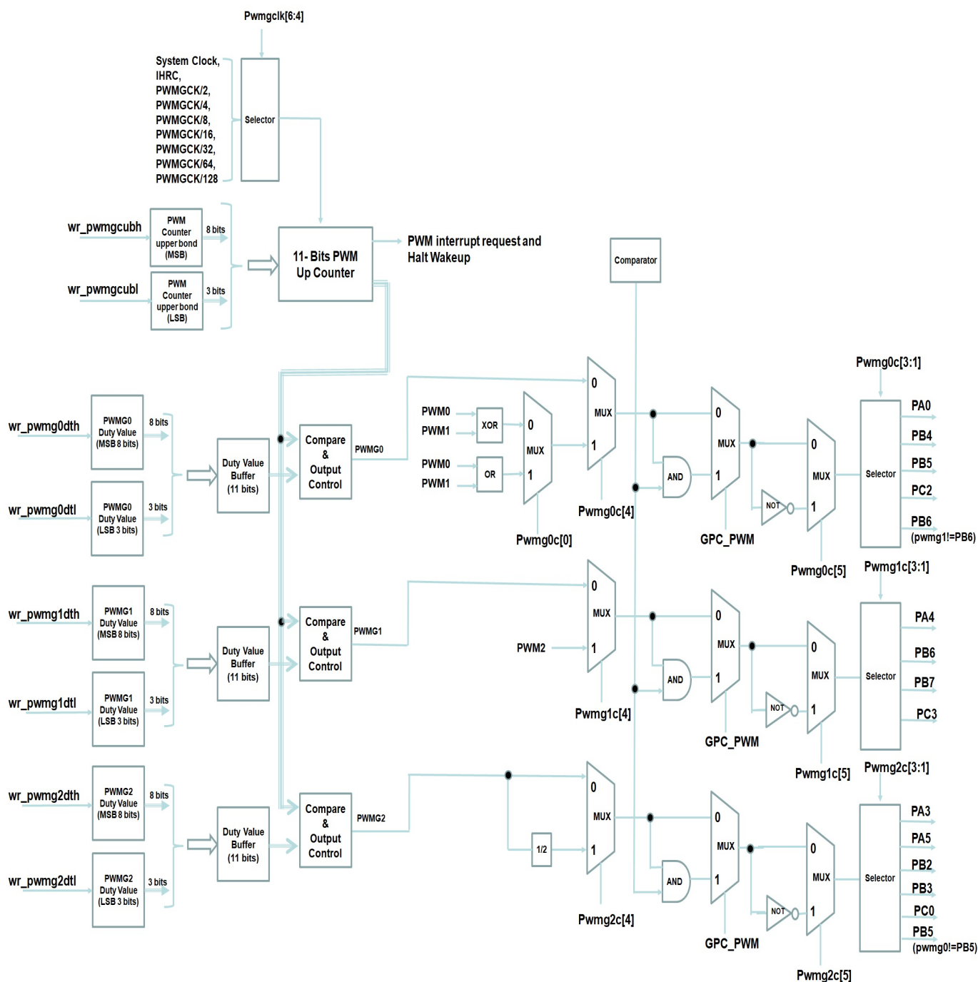
图 15: 整组三路 11 位 PWM 生成器硬件框图
